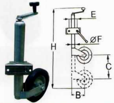
Koło podporowe pneumatyczne
