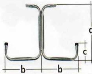
Hak sufitowy typu „T”
