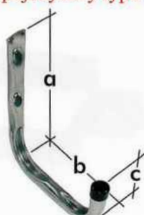
Hak pojedynczy typu „U”
