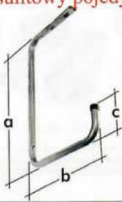
Hak sufitowy pojedynczy
